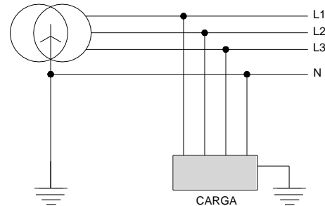
Figura 4 - Esquema TT
