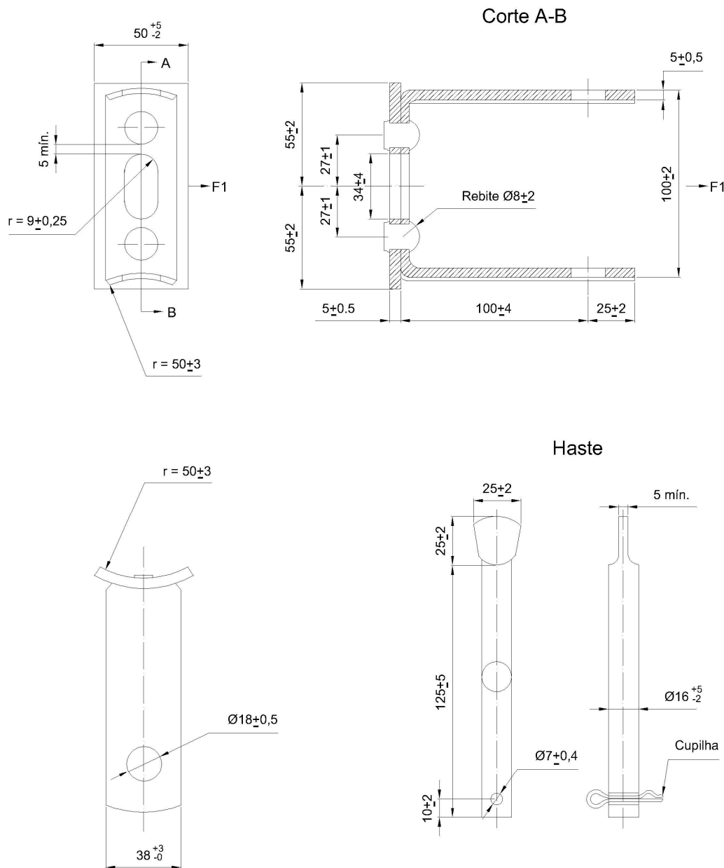
Figura 6 - Desenho dimensional armação secundária de 1 estribo
