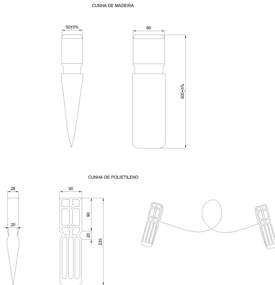
Figura 5 - Desenho dimensional cunha separadora de fases
